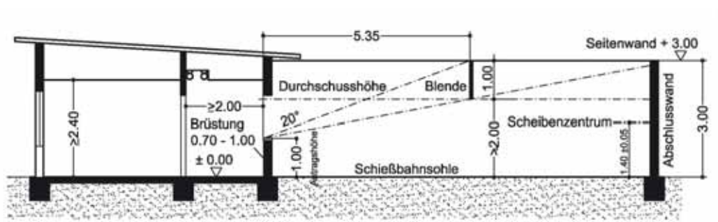
Abbildung 3.2.2 Längsschnitt eines offenen DL-Schießstandes (Prinzip)
