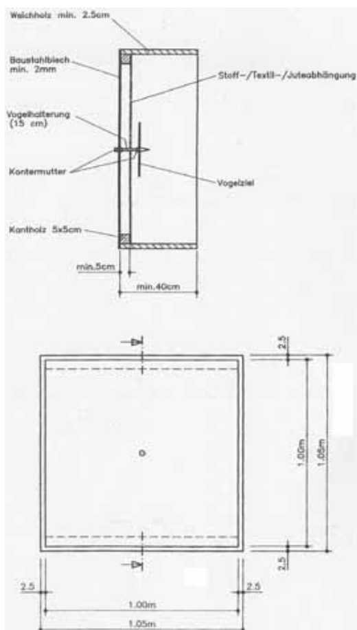
Abbildung 7.9.3 Geschosfang für DL-Waffen auf Vogelschießständen
