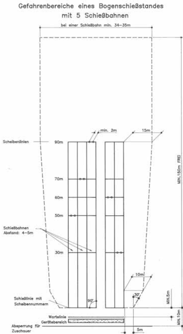
Abbildung 8.3.2 Abmessungen eines Bogenschießstandes
