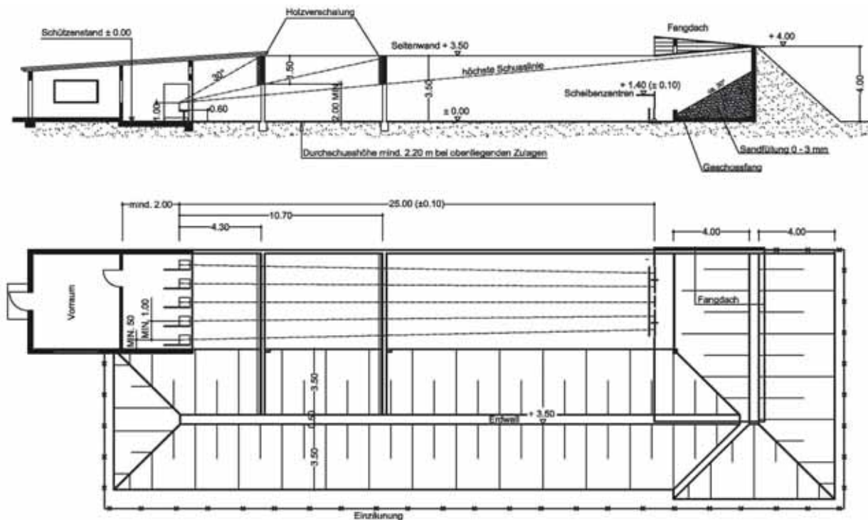
Abbildung 4.8.1 25-m-Schießstand
