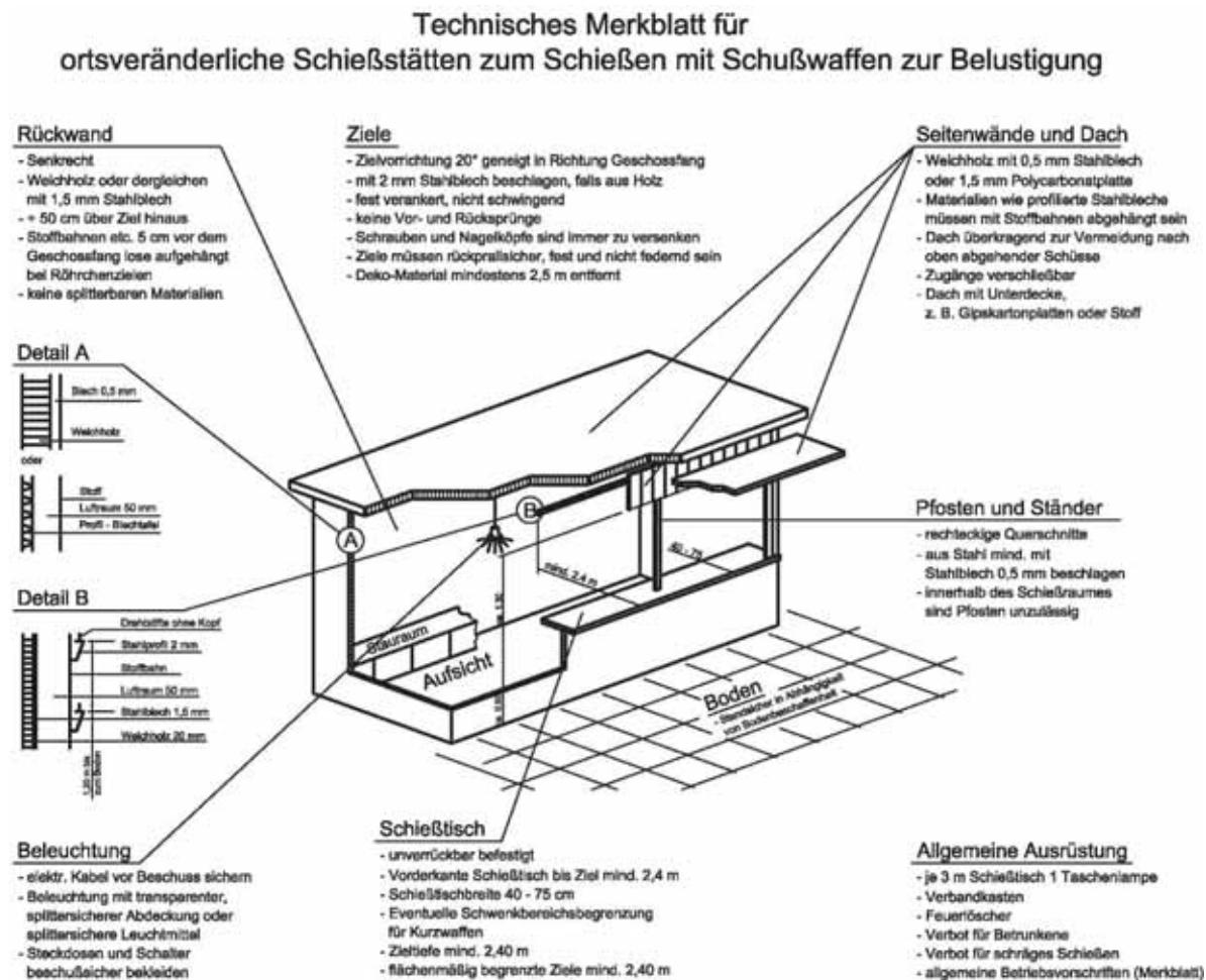
Abbildung 6.5.5 Technisches Merkblatt „Schießbuden“
