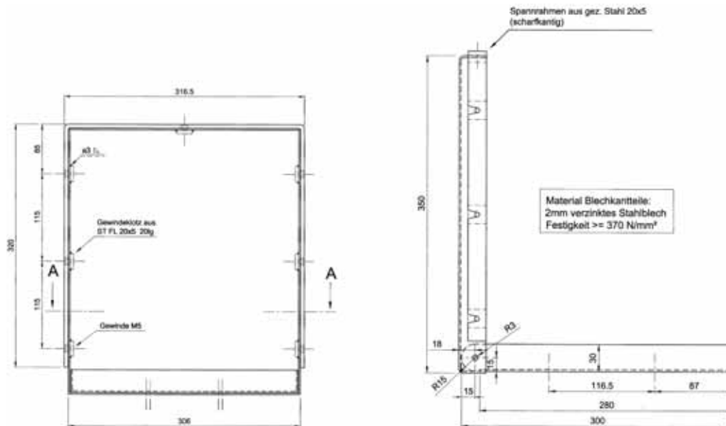
Abbildung 6.4.6.4 Abmessungen eines Field-Target-Geschossfanges
